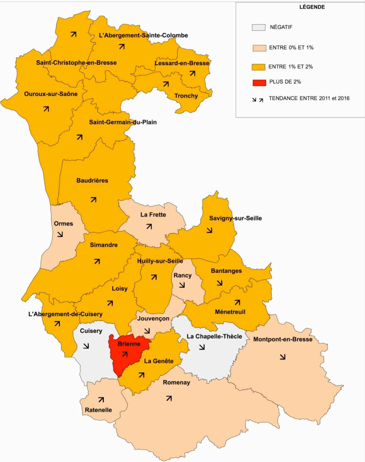
Taux de croissance démographique annuel moyen entre 1999 et 2016
